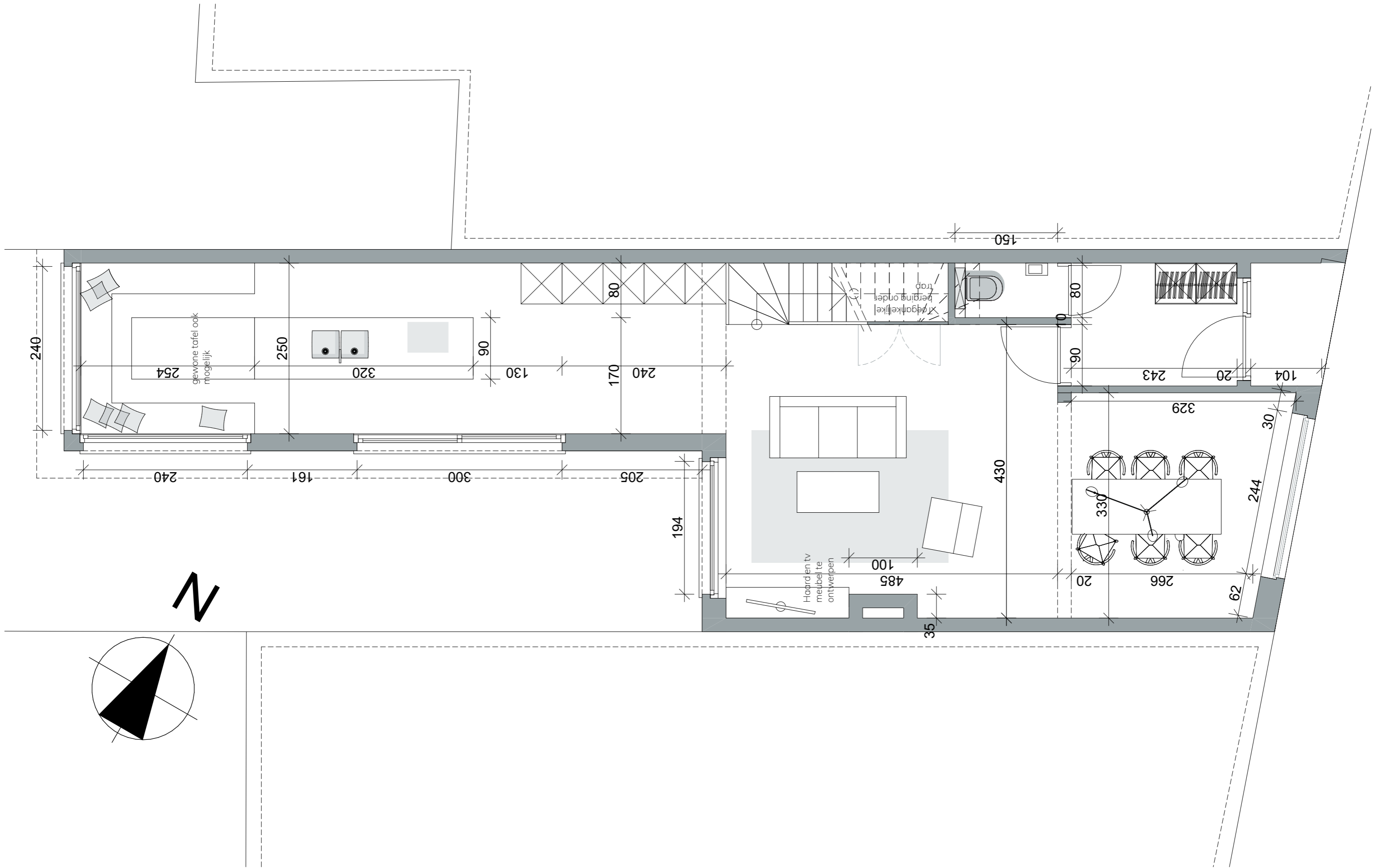
Plan schaal 1:50
